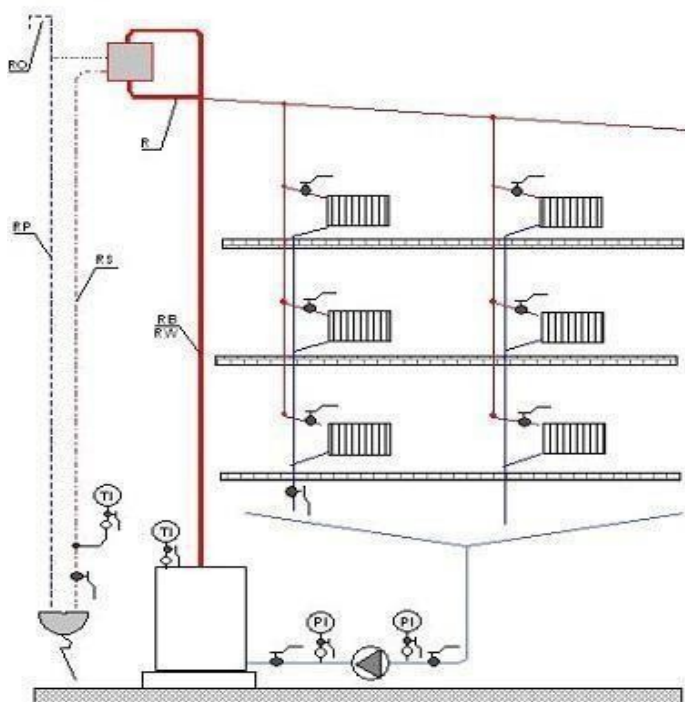
Obr. 2 Schéma ochrany pro systém ohřevu vody s jedním kotlem, čerpadlo instalované ve vratném potrubí RO-ventilační potrubí RP-přepadové potrubí RW-expanzní potrubí RS-signální potrubí RB-bezpečnostní potrubí.
