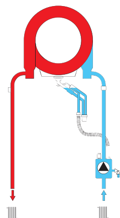
VODNÁ SCHÉMA mod. 45
