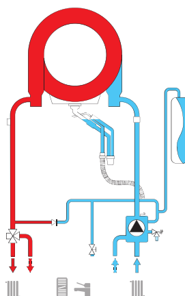
VODNÁ SCHÉMA mod. 18-25-35
